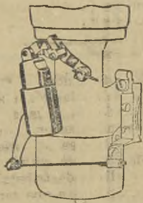
Bomba de accellerção do carburador
